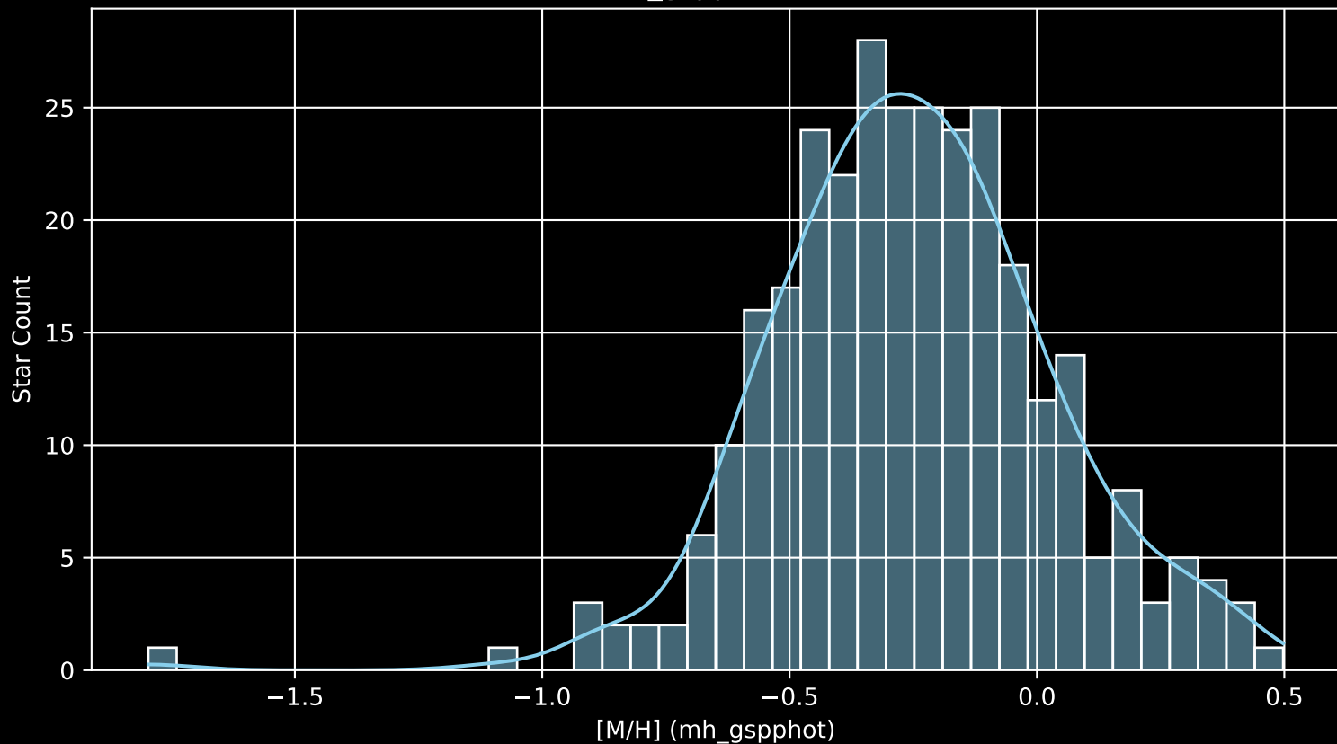
GALAH DR4 Field: [363] [M/H] (mh_gspphot) (n= 306)
