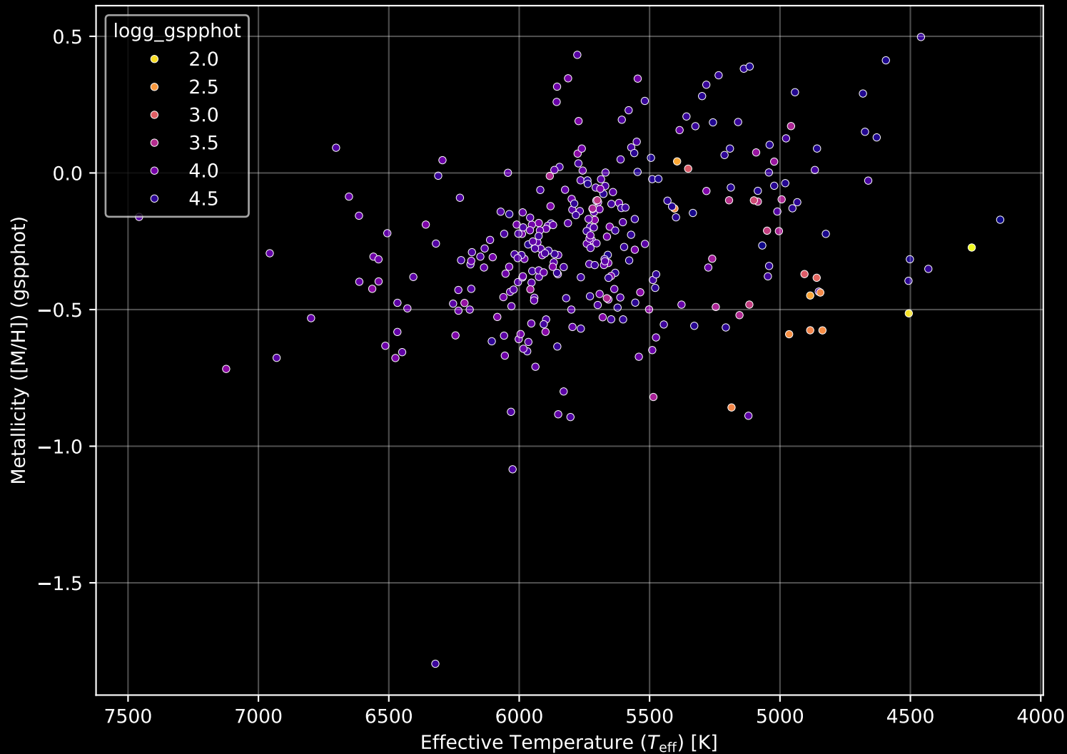
GALAH DR4 Field: [363] Stellar Population Parameters (n= 306)
