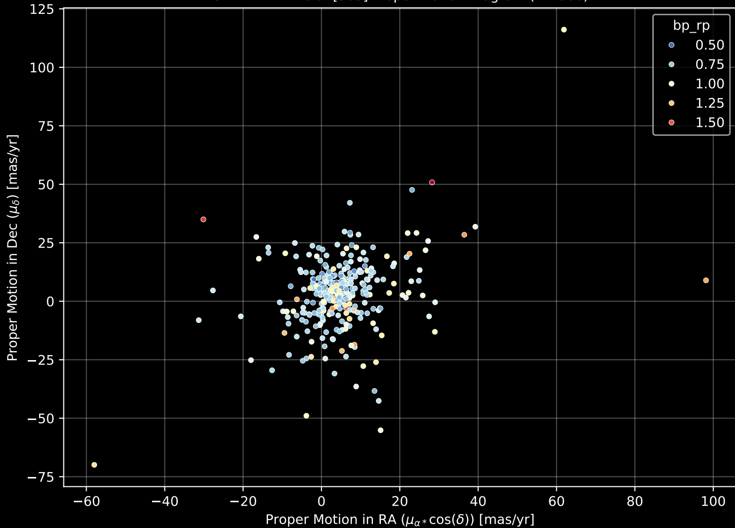
GALAH DR4 Field: [363] Proper Motion Diagram (n= 306)
