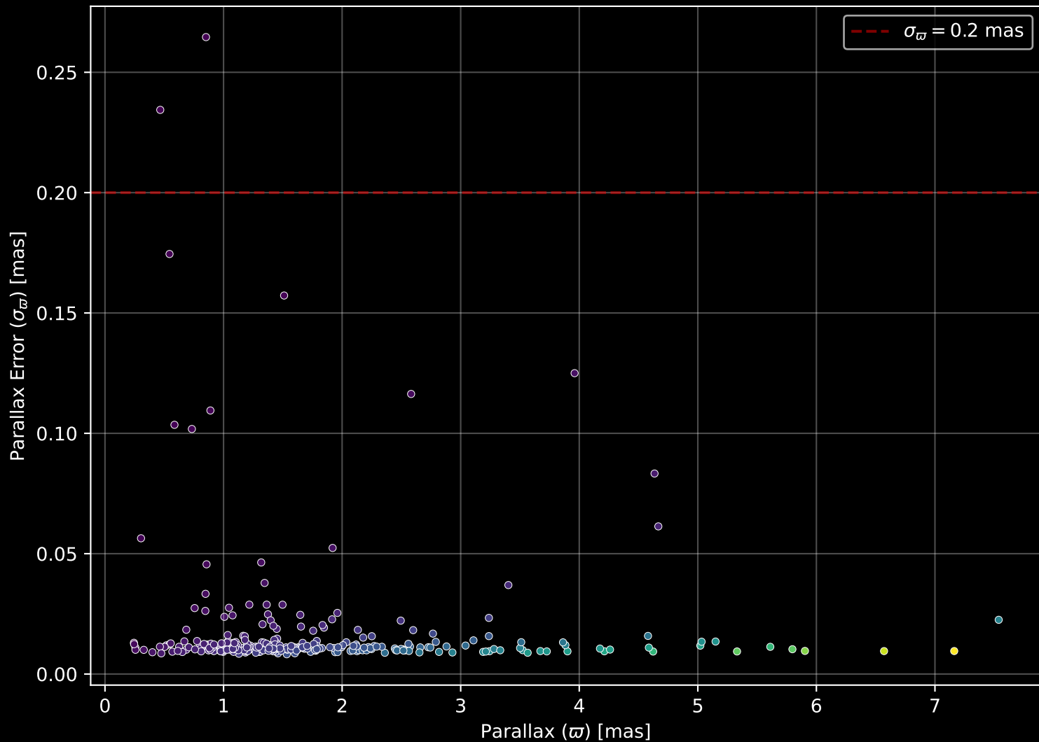
GALAH DR4 Field: [363] Parallax Quality (n= 306)
